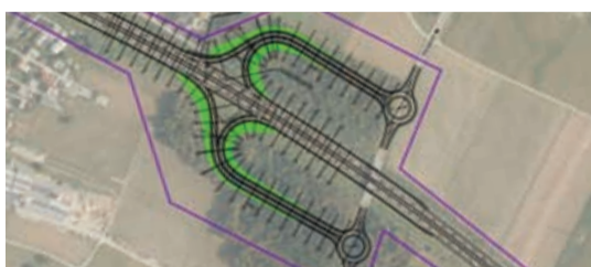
Izvoz AC Kranj-sever – S številnimi aktivnostmi smo uspeli dokazati državi, da je nov, nujno potreben avtocestni priključek ustrezen.
